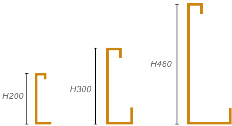
Doorsnede van de keerwanden
